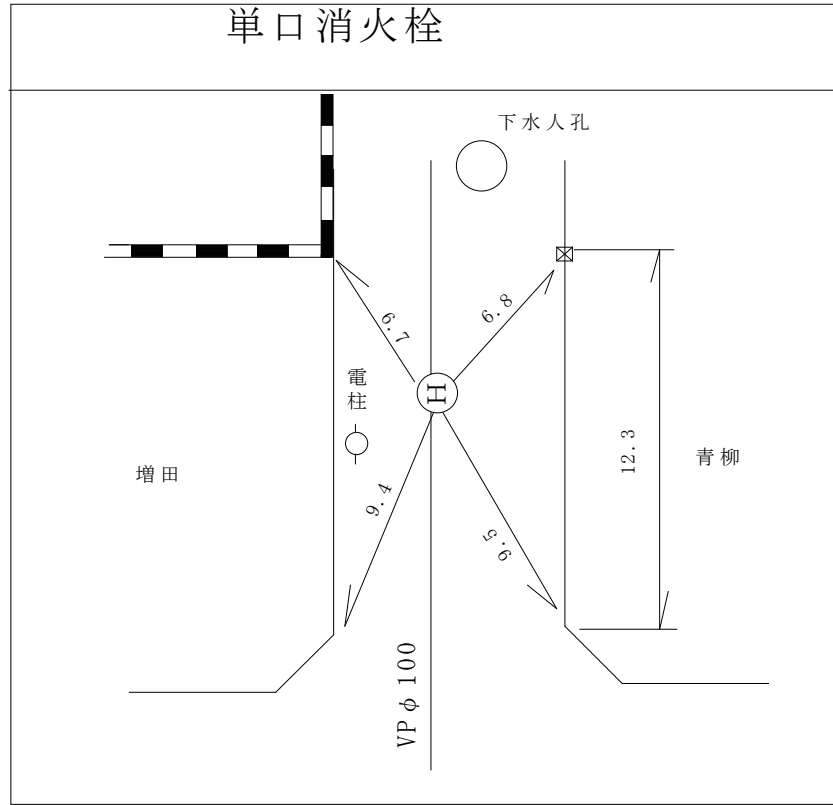
図ー2 オフセット標準図
