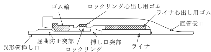
図一5.13 異形管接合（ライナ使用）図
