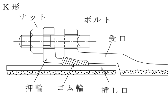
図ー 5.1 K 形管の接合
