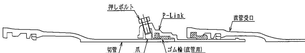
図 5.21 GX 形 P-Link
