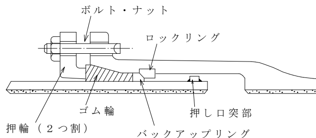
図一5.8 S II 形管の接合
