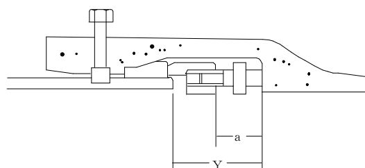
図ー5.7 胴付間隔及び締付け完了時の押輪と受口底部の間隔
