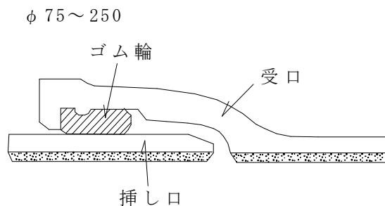
図一5.2 T形管の接合
