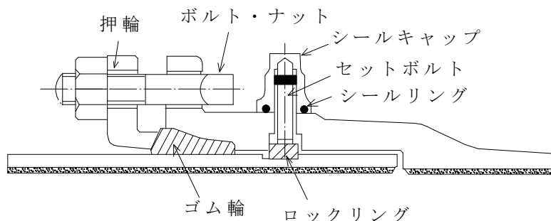
図一 5.3 K F 形管の接合
