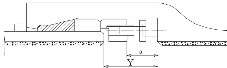
図ー5.5 胴付間隔及び締付け完了時の押輪と受口底部の間隔
