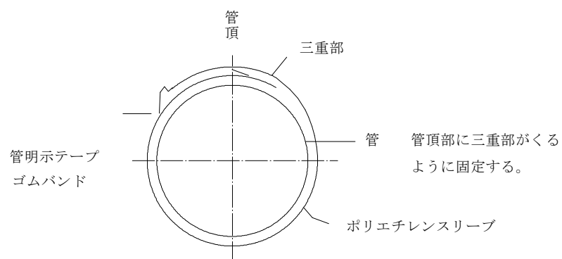
図ー 1 ポリエチレンスリーブ固定方法
