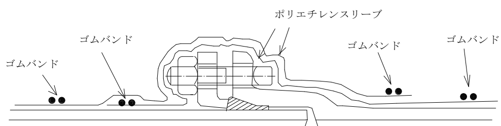
図ー 2 継手部分の施工方法
