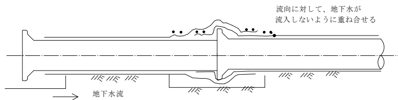
図ー３ 傾斜配管におけるスリーブの施工方法
