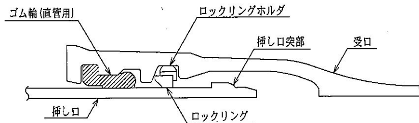
図 5.19 GX形直管の接合
