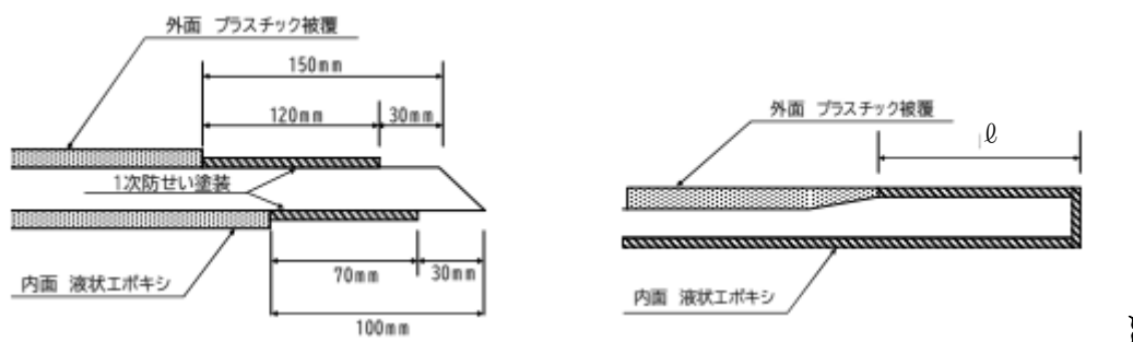
図 6.2 管端内外面塗覆装の仕上げ
