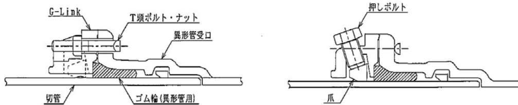
図 5.22 GX 形 G-Link
