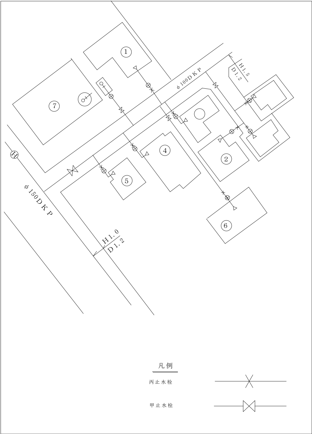
图一 3 给水装置图
