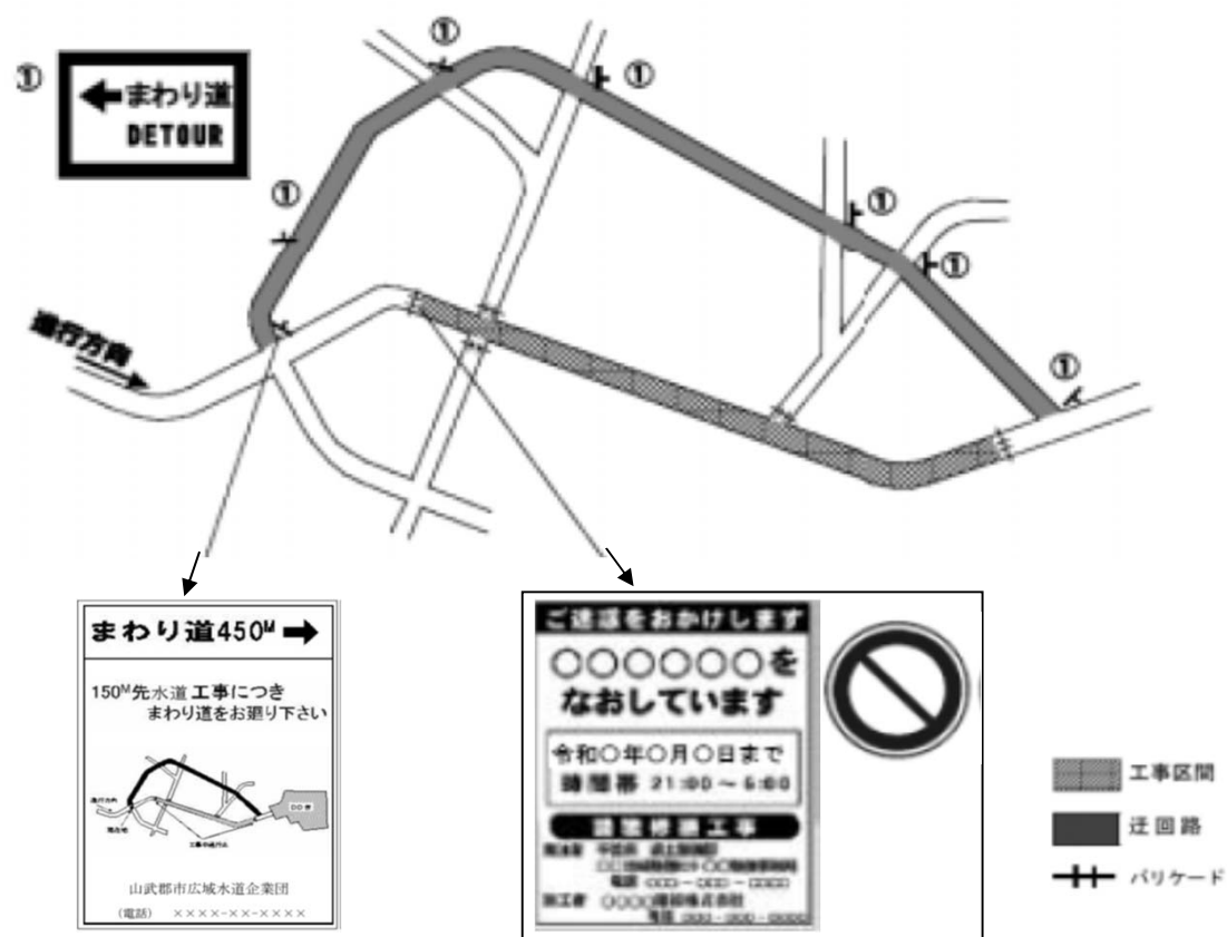
参考（３） 工事中迂回路の表示例（地方部の場合） （進行方向に対する標識の設置例を示す）
