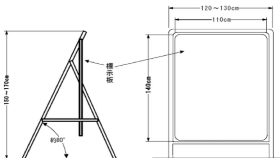
参考（４） 設置方法の一例
