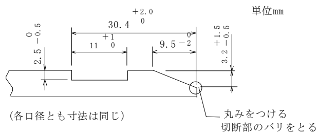
図一5.14 挿し口加工寸法
