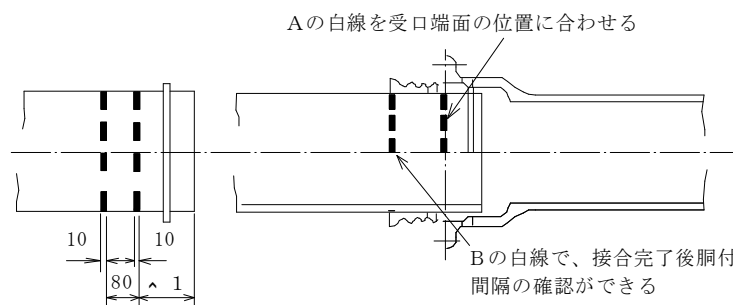
図 5.9 受け口・挿し口の挿入完了(単位:mm)
