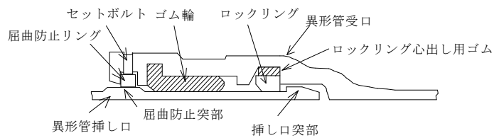
図一5.12 異形管接合図
