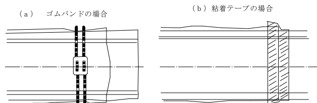
図ー４ スリーブの固定方法
