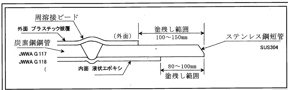
図 8.2 管端内外面塗覆装の仕上げ
