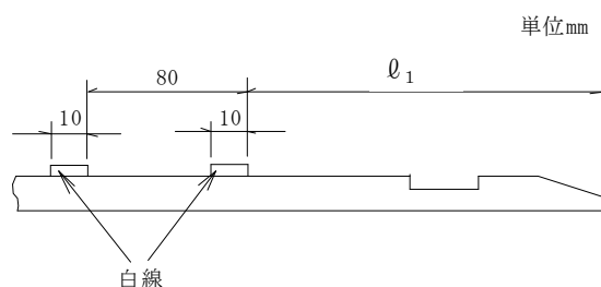
図一5.15 白線表示位置
