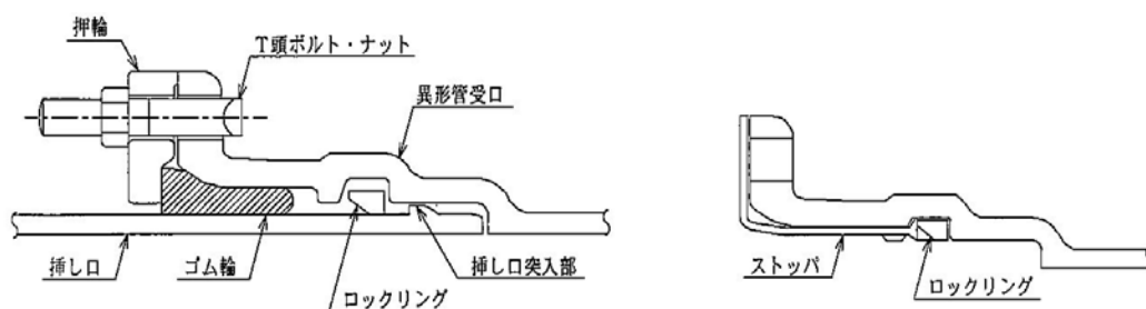
図 5.20 異形管の接合
