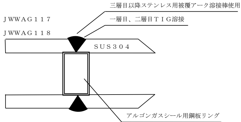
図 8.1 鋼管部と開先部の溶接
